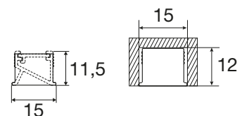
Kaleo Einbau flächenbündig
