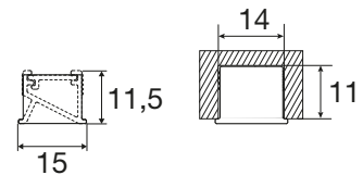
Kaleo Einbau
