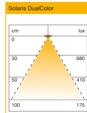
Lichtverteilungsdiagramm
