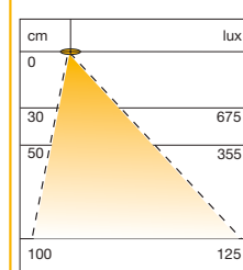
Lugano IR IP44 DualColor
